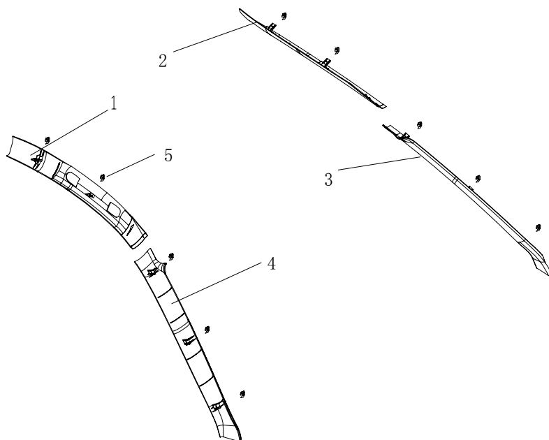
图一 前立柱上装饰板与顶盖装饰板分解图
